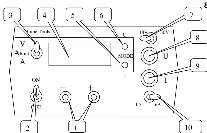
Рис. 1. Передняя панель источника питания
