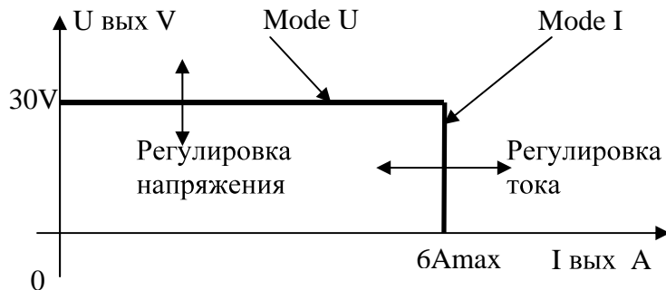
Рис. 2. Вольтамперная характеристика источника питания
