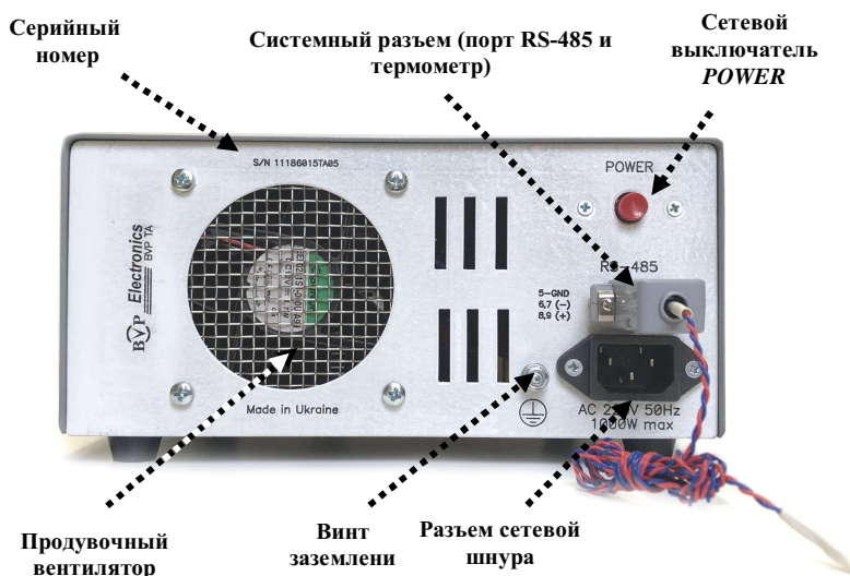
Рис. 4. Задняя панель источника питания
